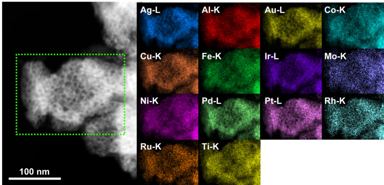
図3 14元素ナノポーラス超多元素触媒のX線マッピング像
