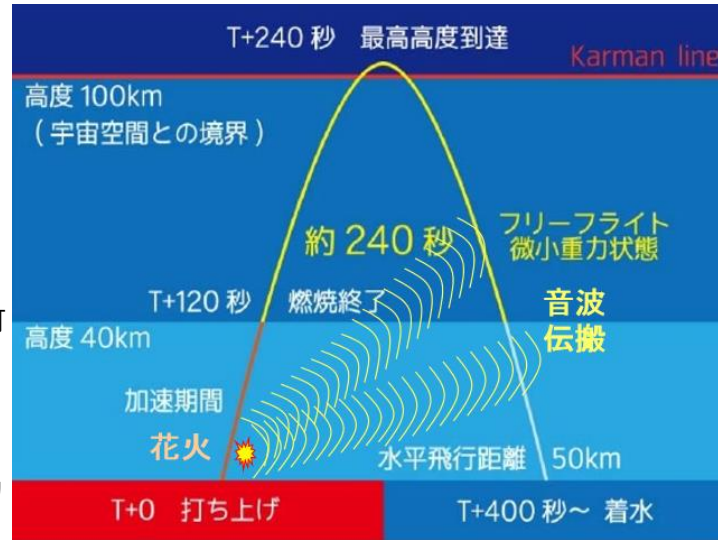
観測ロケット「MOMO2号機」の飛行経路
