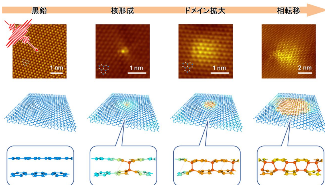
図 1 光誘起相転移の初期プロセス
