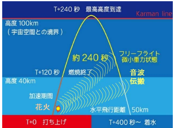
観測ロケット「MOMO2号機」の飛行経路
