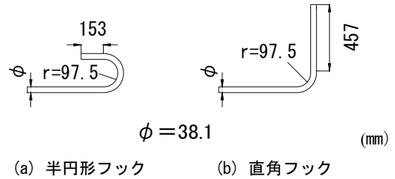
図-2 フックの形状と寸法
