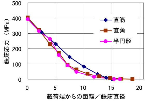
図-8 半円形フック試験体の軸ひずみ分布
