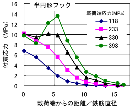
図-11 半円形フック試験体の付着応力分布
