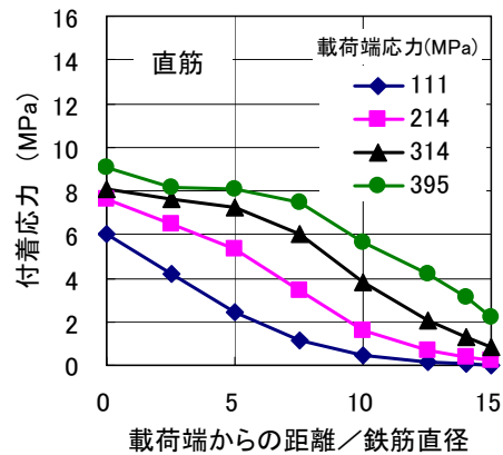
図-9 直筋試験体の付着応力分布
