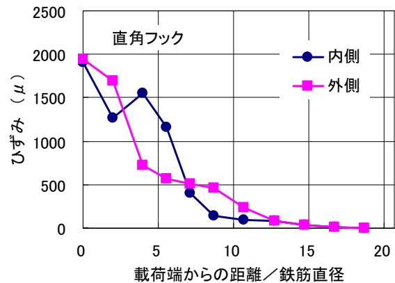
図-5 直角フック試験体における内外のひずみ分布
