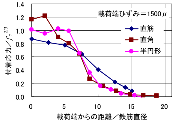
図-13 載荷端ひずみが 1500\mu の時の付着応力分布
