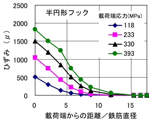
図-7 半円形フック試験体の軸ひずみ分布
