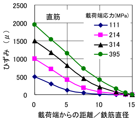
図-4 直筋試験体のひずみ分布
