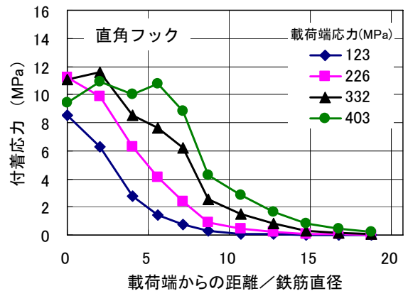
図-10 直角フック試験体の付着応力分布
