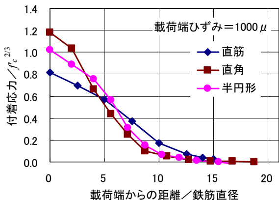
図-12 載荷端ひずみが 1000\mu の時の付着応力分布
