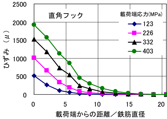
図-6 直角フック試験体の軸ひずみ分布
