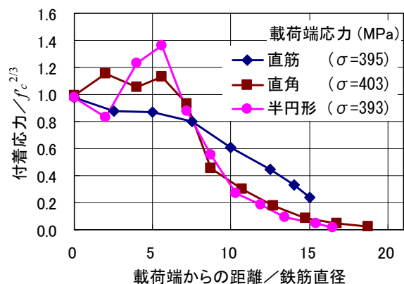
図-14 載荷端応力が約 400MPa の時の付着応力分布
