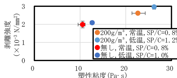
図-3 低温によるフロー値低下を減水剤添加量増で補った場合，粘度と粘着力の上昇量が増粘剤添加により増加
