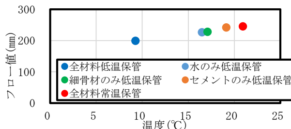
図-4 使用材料の保管温度を反映したモルタルの練り温度とフロー値との関係
