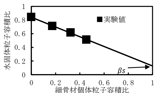
図-1 外挿して相対フロー面積比が 0 となる細骨材個体粒子容積比を細骨材の拘束水比 \beta_s と定義して求めた
