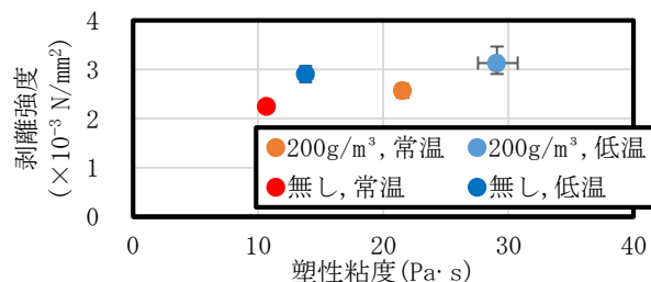
図-2 新型増粘剤の添加が低温によるペーストの粘度と粘着力の上昇量を大きくした
