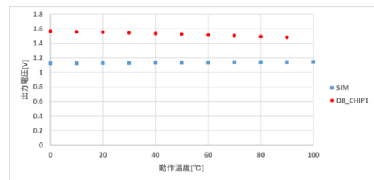
図 3.2 BGR 回路の温度特性
