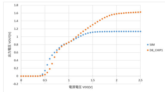
図 3.1 BGR 回路の電源電圧特性
