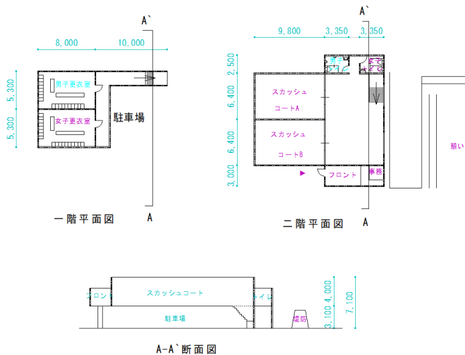
図8 スカッシュ施設図面
