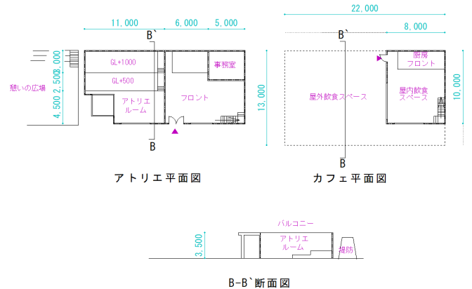
図18 アトリエカフェ図面
