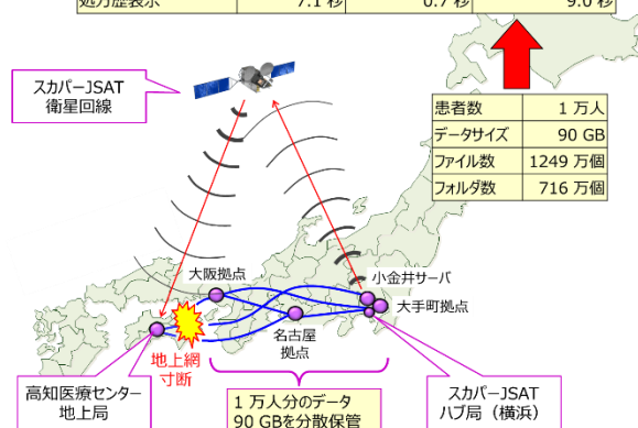
図1 実証実験に用いたネットワーク接続図と性能評価結果
